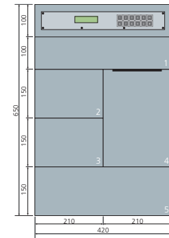
Konfigurationsbeispiel Mono 420-5 EZ
